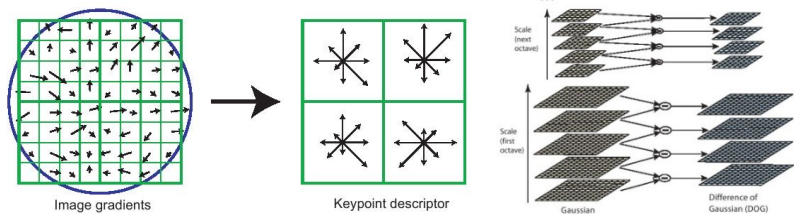
SIFT
