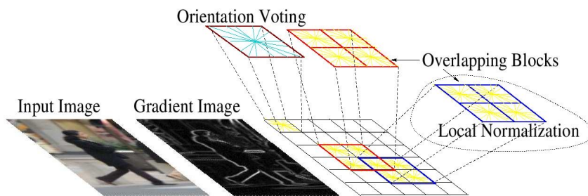
HoG
